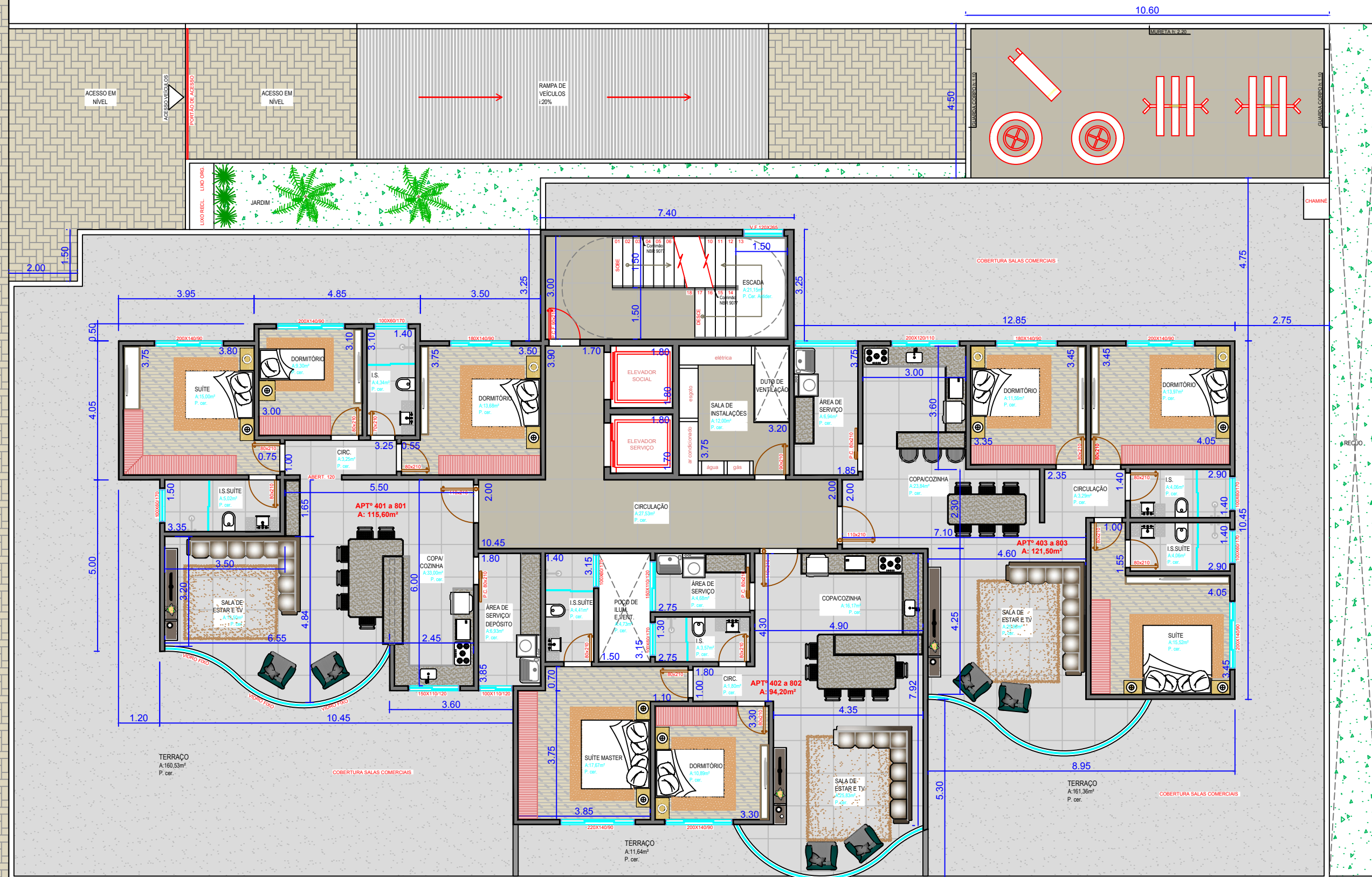
PLANTA BAIXA-TIPO(X5) SEM ESCALA
