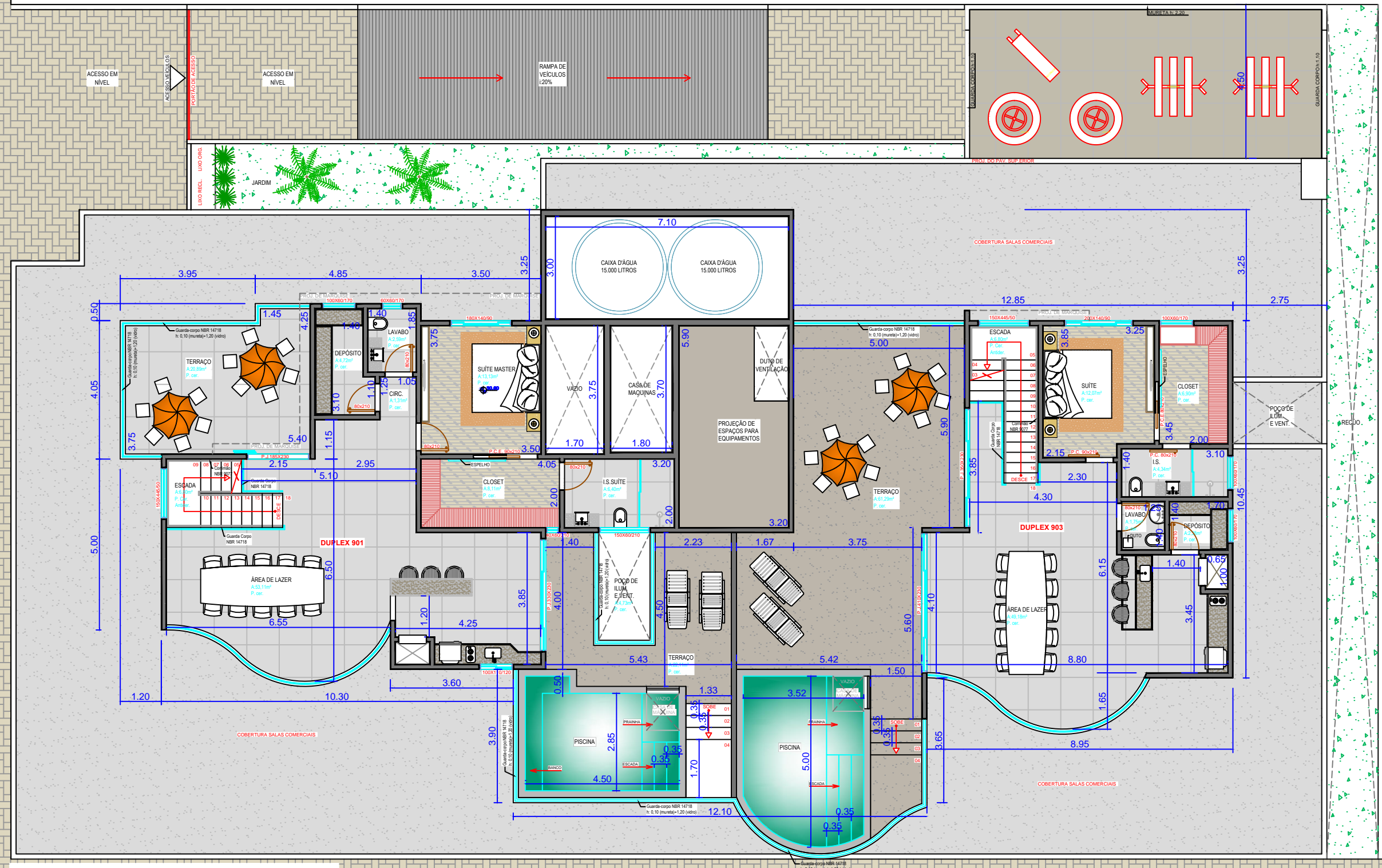
PLANTA BAIXA-SUPERIOR DUPLEX SEM ESCALA
